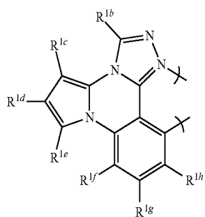
gs3-3
