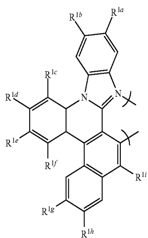
gs1-15
