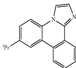
es6 ligand
