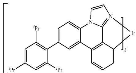
es18
