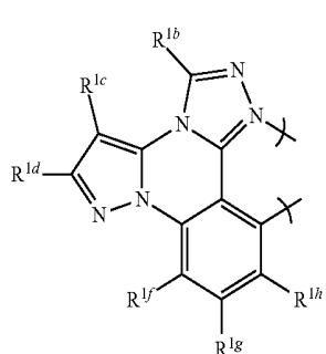
gs3-11
