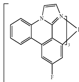
es5
