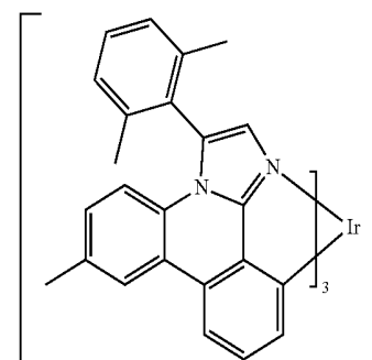
es20
