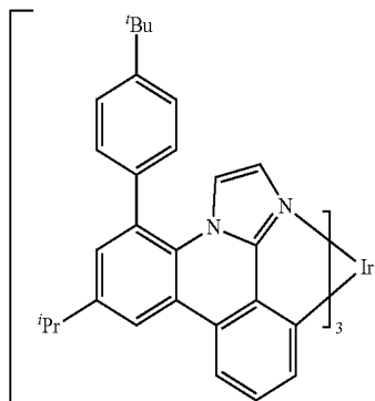
es17
