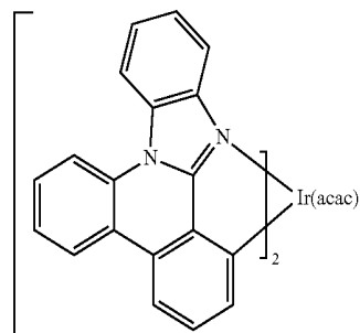
es2
