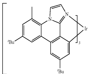
es19
