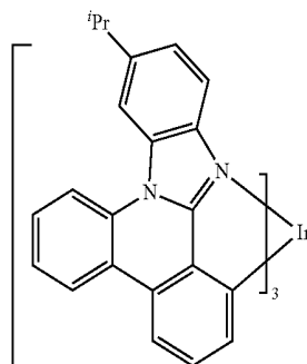
es4
