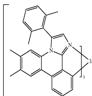
es21
