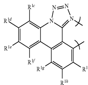
gs1-5
