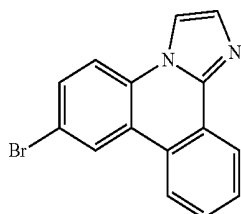
es13-il
