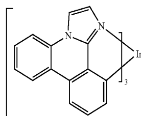
es1
