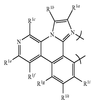
gs1-18
