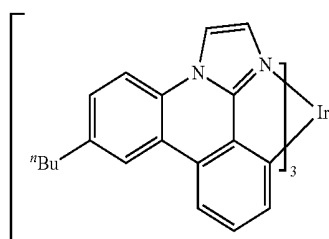
es15
