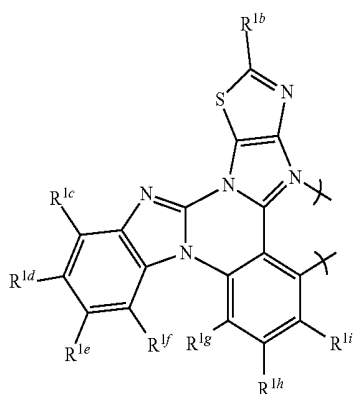
gs3-22
