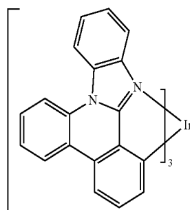
es3
