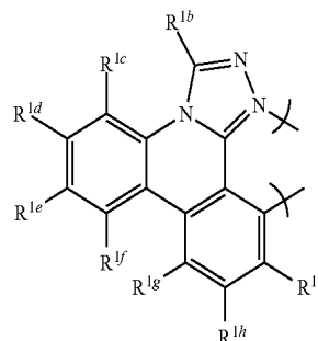
gs1-2
