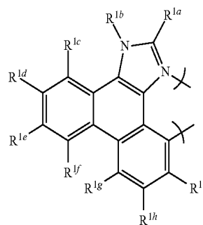
gs1-4
