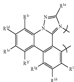
gs1-3
