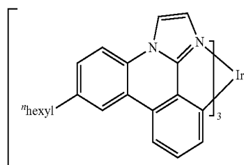
es8
