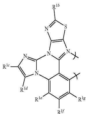
gs3-23
