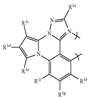
gs3-2
