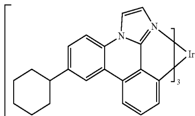
es16
