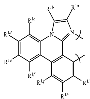
gs1-19
