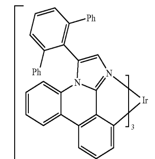
es23
