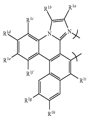
gs1-14
