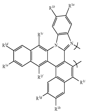
gs1-16
