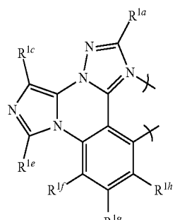
gs3-8
