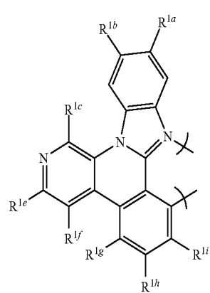
gs1-20
