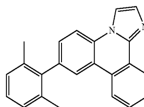
es13 ligand
