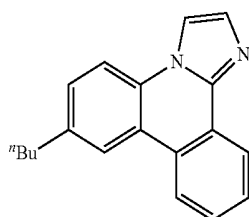
es15 ligand
