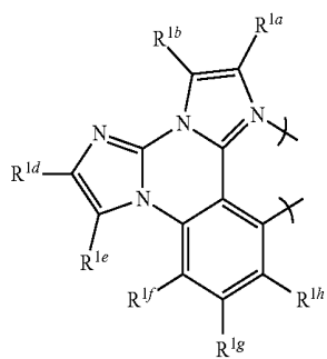
gs3-4
